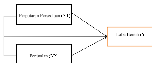
Gambar 2 Kerangka konseptual
